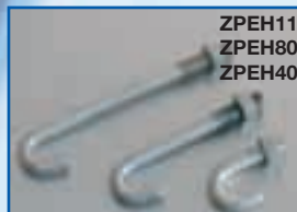
Edelstahl-Hakenschraube M8 inkl. V2A Mutter Längen: 40mm, 80mm, 110mm
