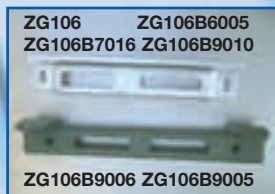
Anschlag mit Schließblech, inkl. Schrauben, Ausführung verzinkt oder Kunststoff, erhältlich in RAL 6005, 7016, 9005, 9006, 9010
